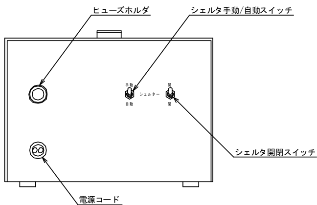
背面図
